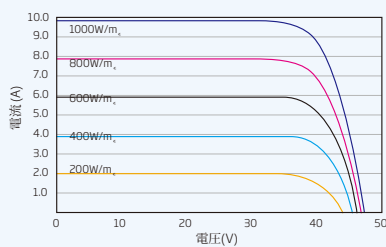
PVモジュール (365W) の I-V 曲線
